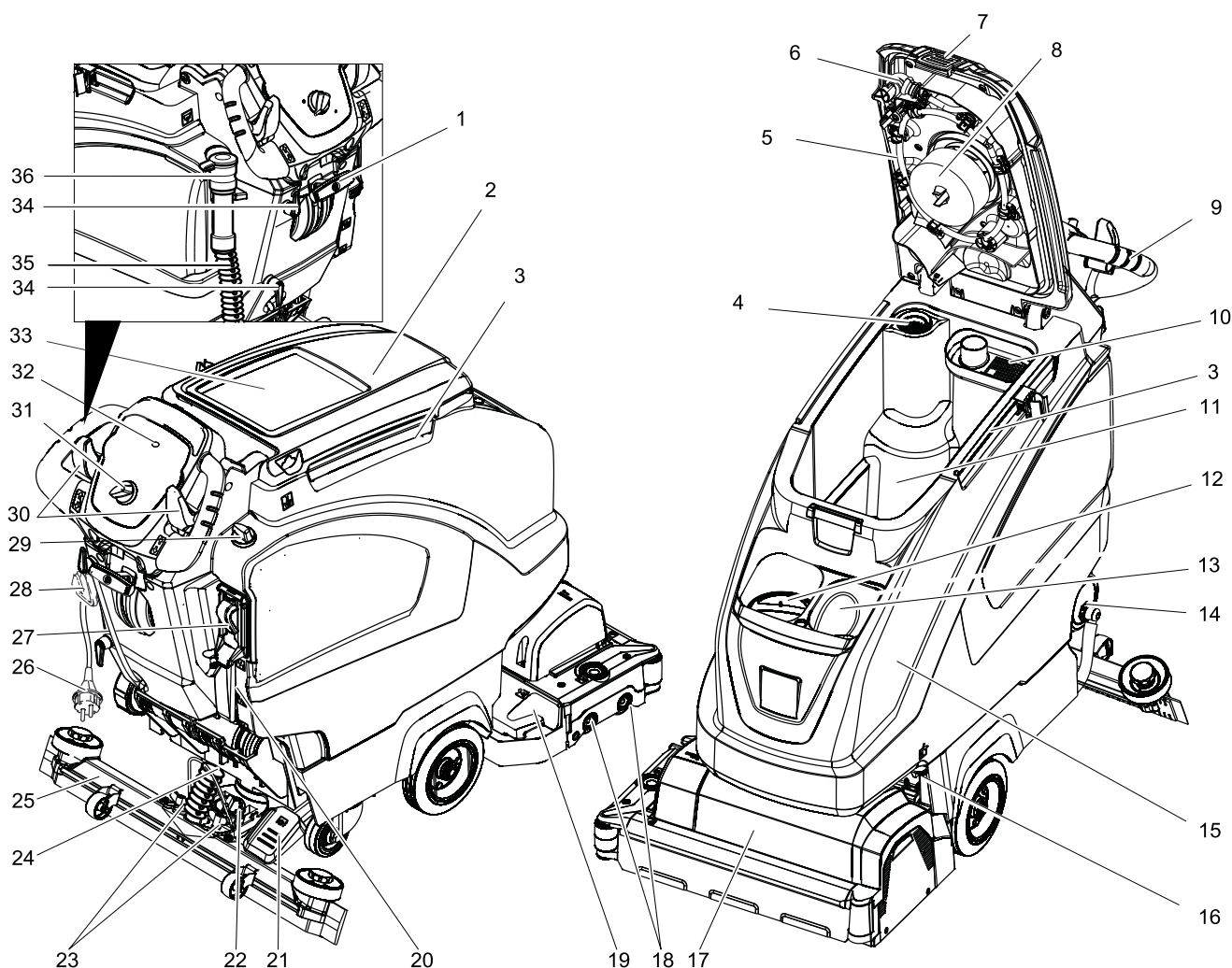
Abbildung Scheuersaugmaschine
